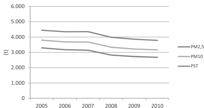
Gráfico 22. Evolución de las emisiones de partículas del sector transporte. Periodo 2005-2010.
