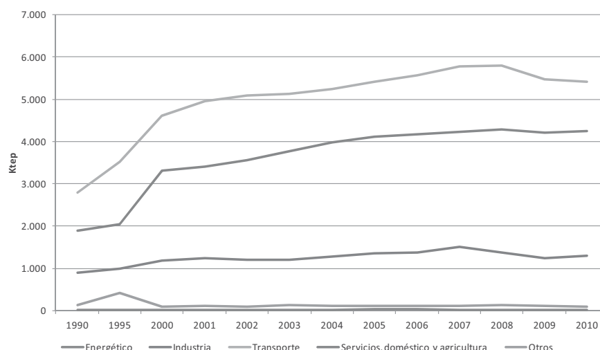
Gráfico 1. Balance energético de la Comunidad de Madrid (ktep) 1 . Años 1990, 1995 y 2000-2010.
