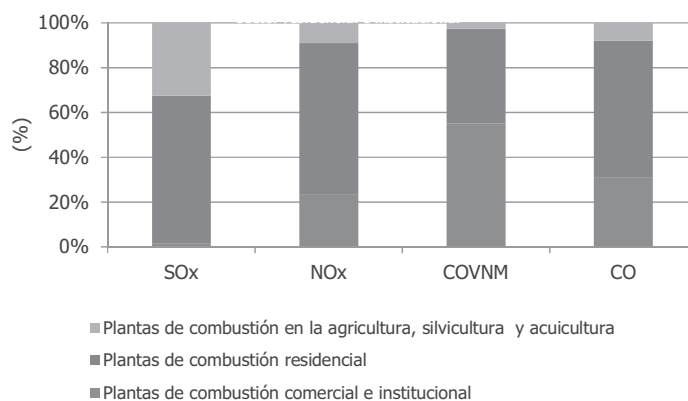
Gráfico 29. Contribución por subsector a las emisiones de sustancias acidificadoras y precursoras del ozono del sector residencial, comercial e institucional. Año 2010.
