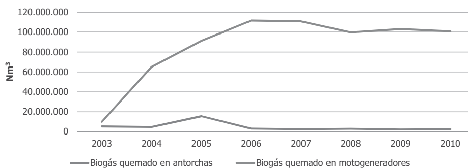
Gráfico 17. Evolución del biogás tratado.
