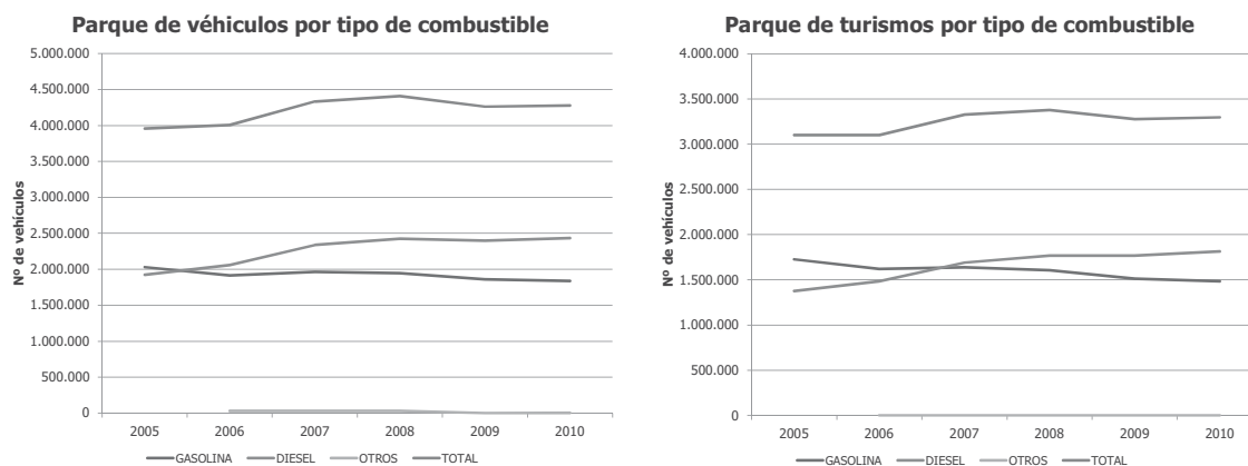
Gráfico 13. Evolución del parque de turismos y del parque total de vehículos por tipo de combustible en la Comunidad de Madrid. Período 2005-2010.
