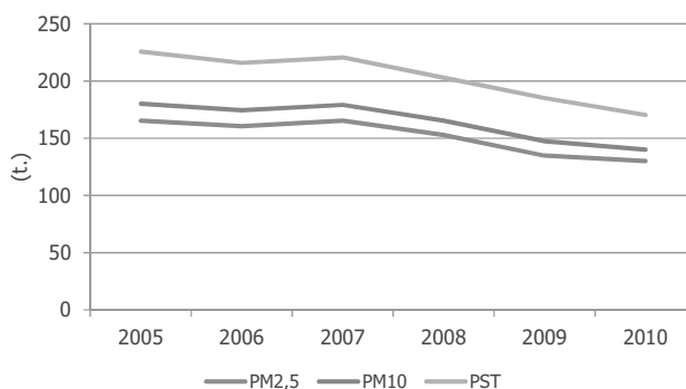
Gráfico 31. Evolución de las emisiones de partículas del sector residencial, comercial e institucional.
