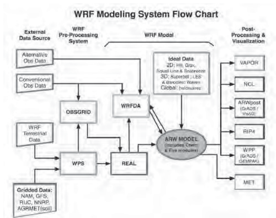
Imagen 4. Representación esquemática de funcionamiento de WRF-ARW
