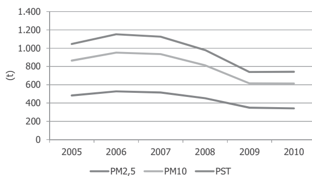
Gráfico 7. Evolución de las emisiones de partículas del sector industrial. Periodo 2005-2010
