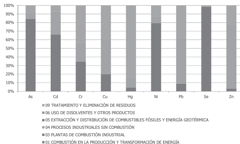
Gráfico 6. Contribución por SNAP a las emisiones de metales del sector industrial. Año 2010
