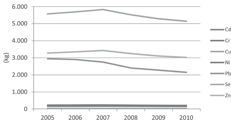
Gráfico 20. Evolución de las emisiones de metales del sector transporte. Periodo 2005-2010.
