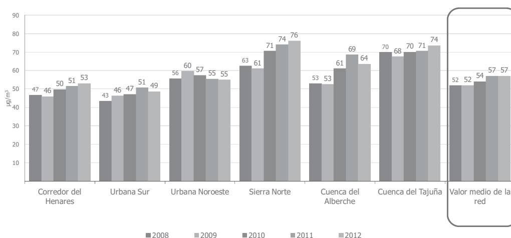
Gráfico 5. Comparativa por zonas de la media anual de ozono. Período 2008-2012
