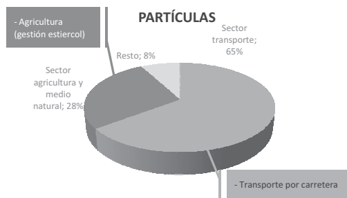
Gráfico 19. Análisis de contribución por sectores a las emisiones de partículas. Basado en inventario del 2010.
