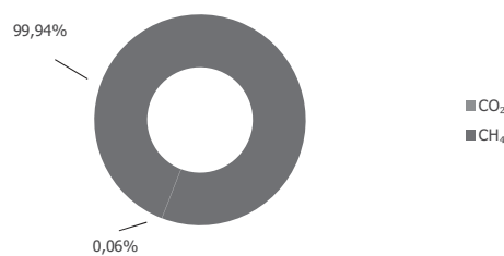
Gráfico 4. Contribución por tipo de GEI a las emisiones del grupo CRF "Energía". Año 2010.
