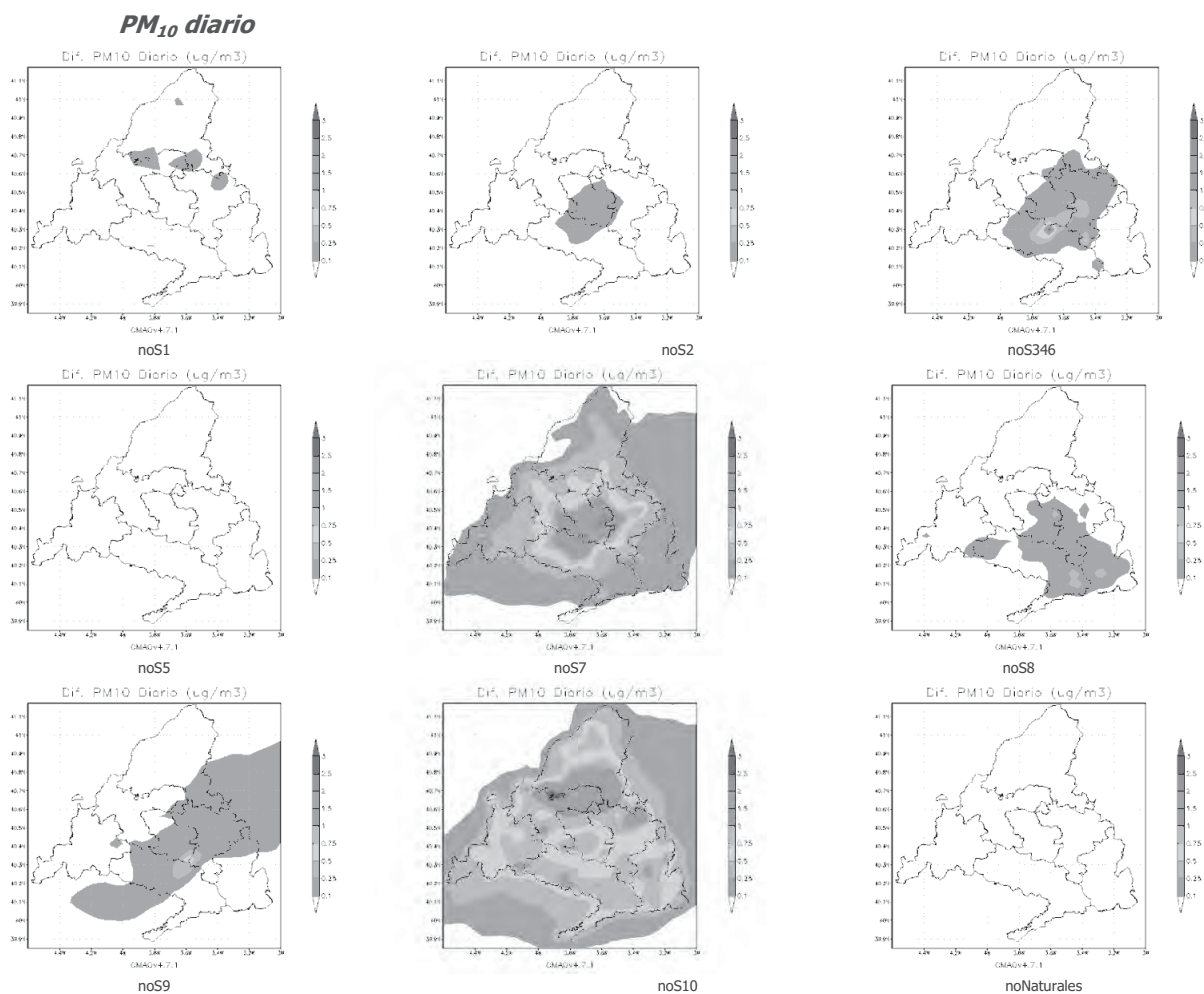
Imagen 10. Diferencias absolutas de los niveles de PM 10 diario en los distintos sectores de emisión respecto al caso base para el dominio d03.
