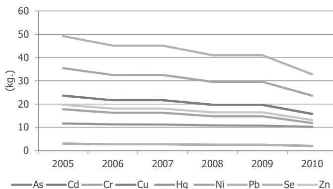
Gráfico 30. Evolución de las emisiones de metales del sector residencial, comercial e institucional. Periodo 2005-2010.
