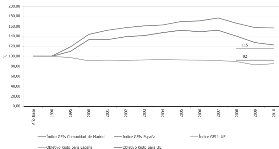
Gráfico 30. Evolución de las emisiones de GEI en la Comunidad de Madrid, España y Unión Europea 10 . Años 1990, 1995 y 2000-2010.
