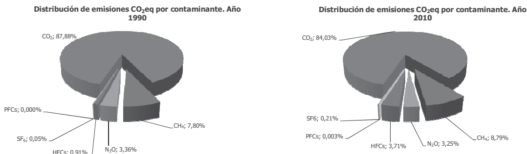
Gráfico 33. Contribución por tipo de GEI a las emisiones totales. Años 1990 y 2010.
