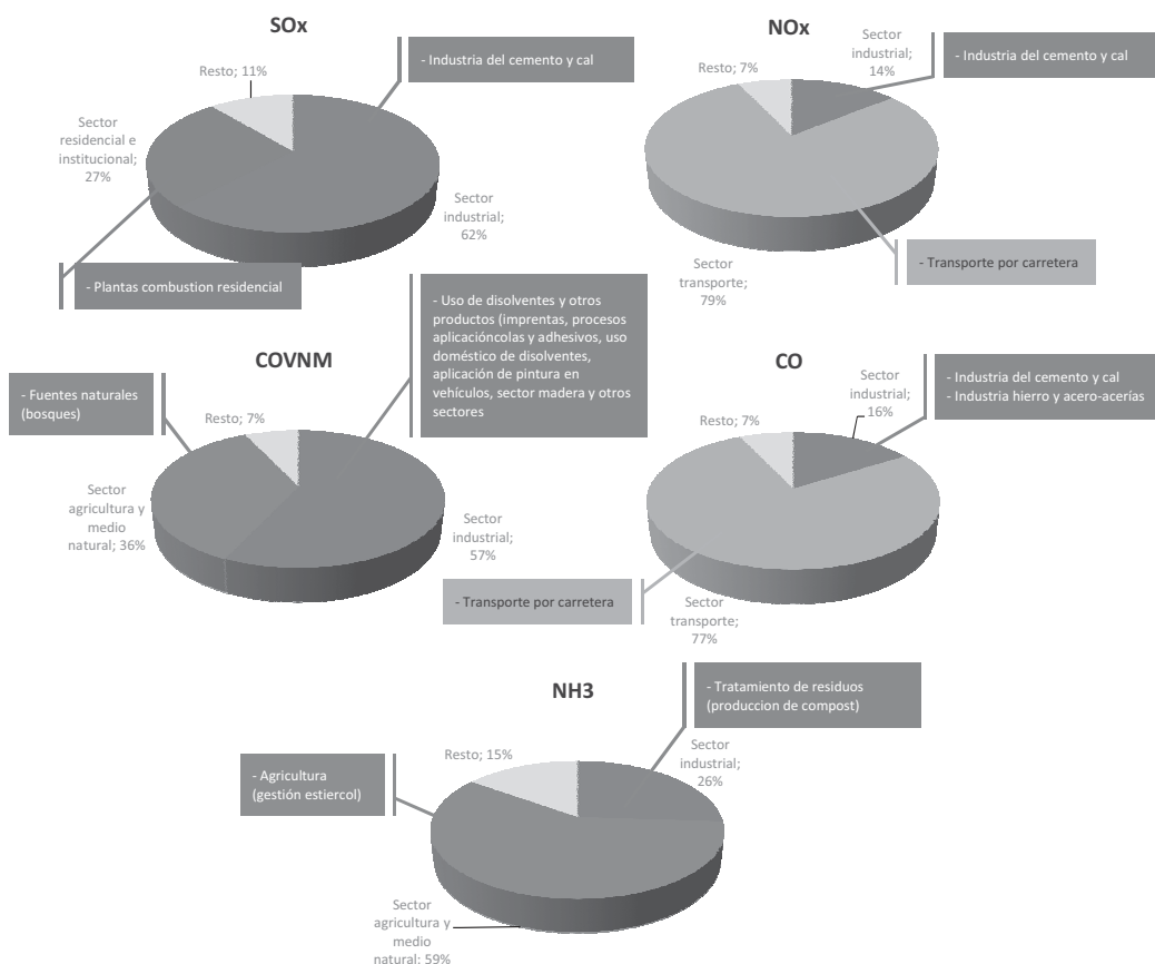
Gráfico 11. Análisis de contribución por sectores a las emisiones de sustancias acidificadoras y precursoras de ozono. Basado en el inventario del año 2010.
