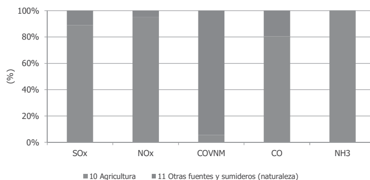
Gráfico 37. Emisiones de sustancias acidificadoras y precursoras del ozono del sector agricultura y medio natural. Año 2010.
