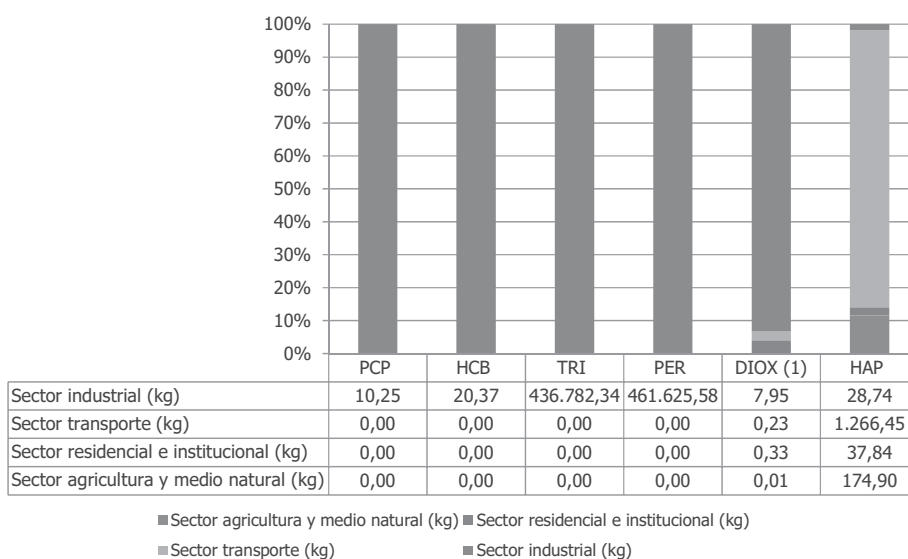
Gráfico 21. Contribución por sectores a las emisiones de compuestos orgánicos persistentes. Año 2010.
