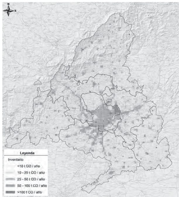
Imagen 3. Inventario de emisiones de CO. Año 2010.
