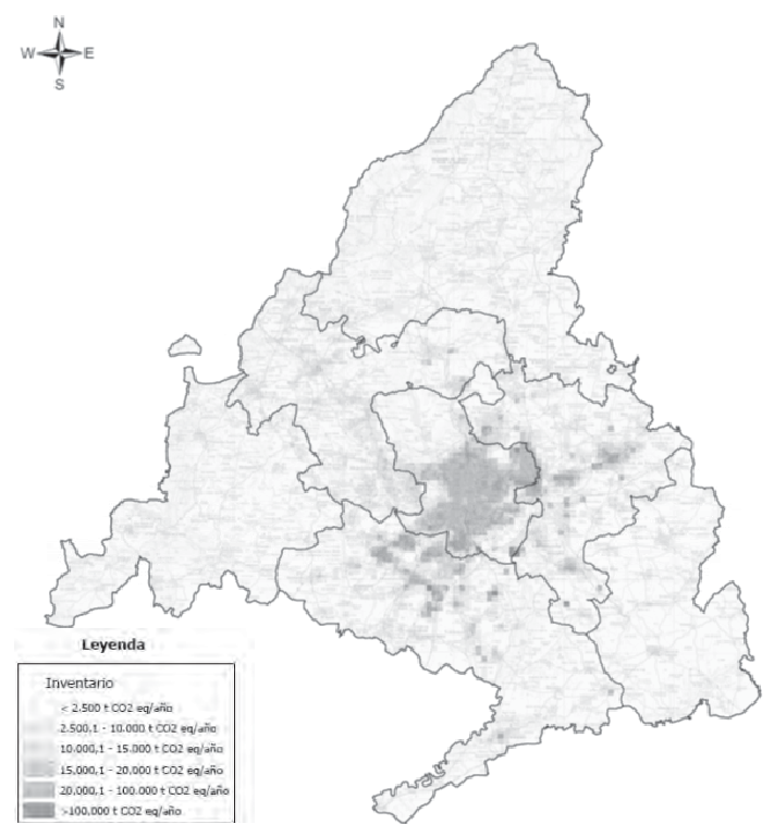
Imagen 11. Inventario de emisiones de GEIs (CO 2 eq). Año 2010.
