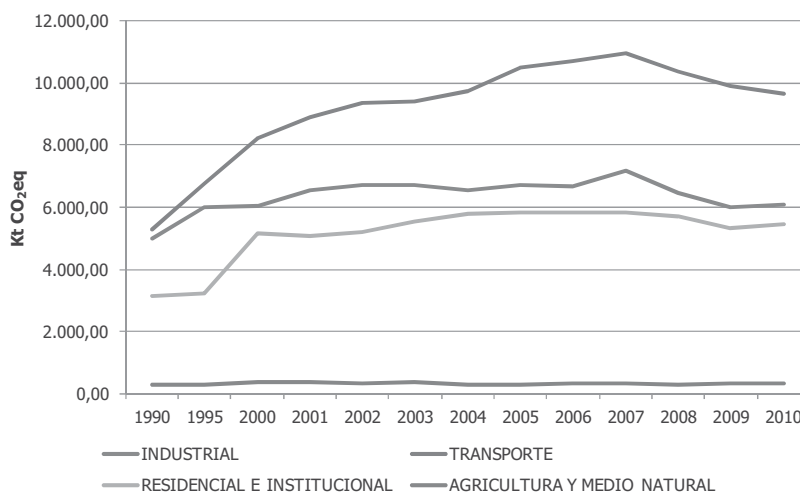
Gráfico 35. Evolución de las emisiones de GEIs por sectores. Año 1990, 1995 y 2000-2010.
