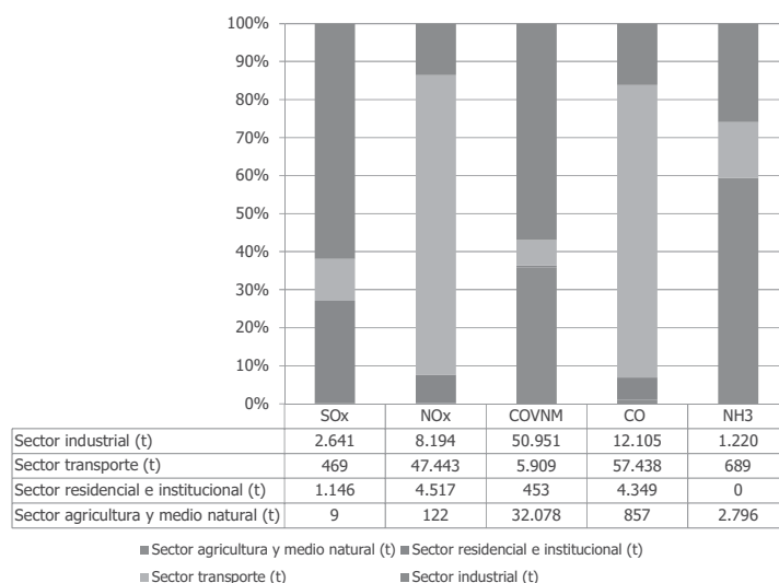
Gráfico 10. Emisiones de sustancias acidificadoras y precursoras del ozono por sectores. Año 2010.
