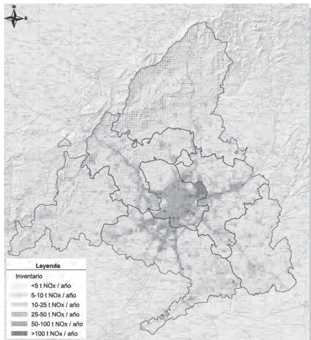
Imagen 2. Inventario de emisiones de NO x . Año 2010.
