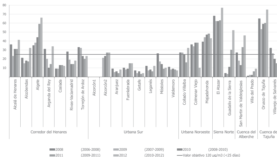
Gráfico 6. Superaciones por estación del valor objetivo para la protección de la salud para ozono. Periodo 2008-2012.
