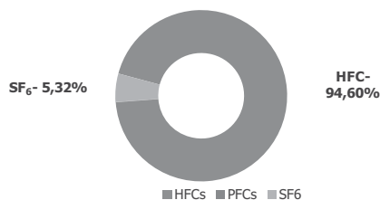
Gráfico 8. Contribución por tipo de GEI a las emisiones del grupo CRF- "Procesos industriales". Año 2010.
