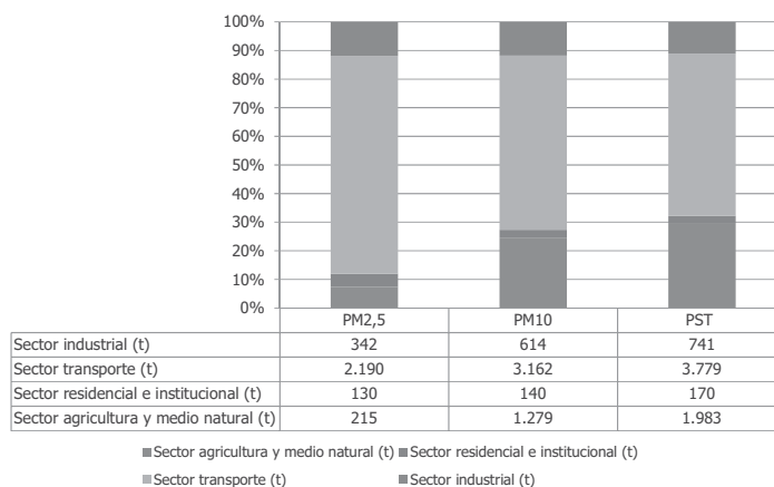
Gráfico 18. Contribución por sectores a las emisiones de partículas. Año 2010.
