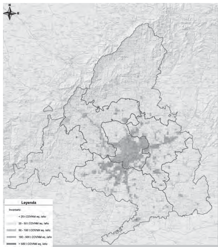
Imagen 5. Inventario de emisiones de precursores del ozono. Año 2010.
