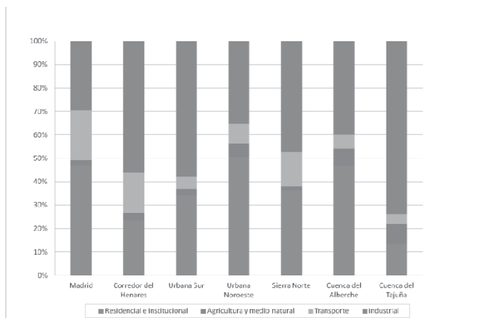
Gráfico 29. Resultados del análisis de contribución de fuentes en las diferentes zonas de calidad del aire para los niveles de SO 2 máx 1-h.
