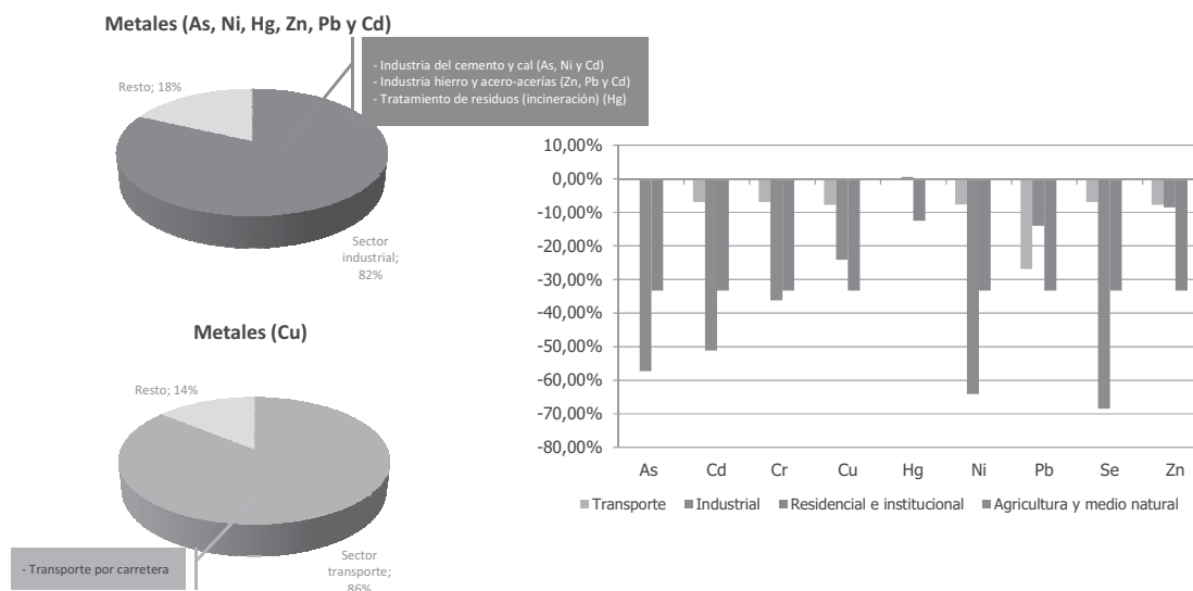
Gráfico 16. Análisis de contribución por sectores a las emisiones de metales. Basado en inventario del 2010.
