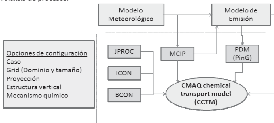
Imagen 9. Esquema de funcionamiento básico del modelo CMAQ. Fuente: www.cmaq-model.org
