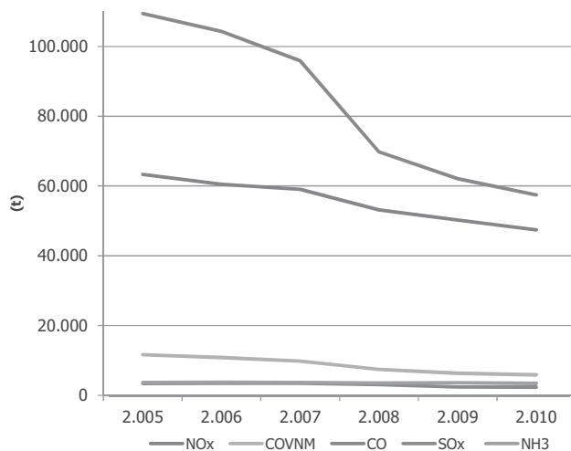
Gráfico 16. Evolución de las emisiones de sustancias acidificadoras y precursoras del ozono del sector transporte. Periodo 2005-2010.
