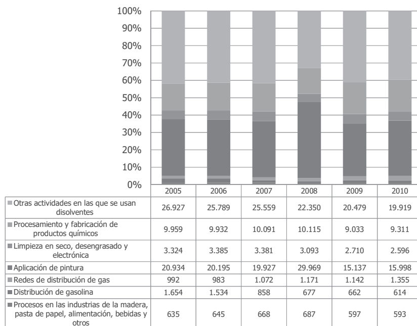
Gráfico 4. Reparto de las emisiones de COVNM del sector industrial. Año 2010
