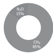
Gráfico 13. Contribución por tipo de GEI a las emisiones del grupo CRF "Agricultura". Año 2010.
