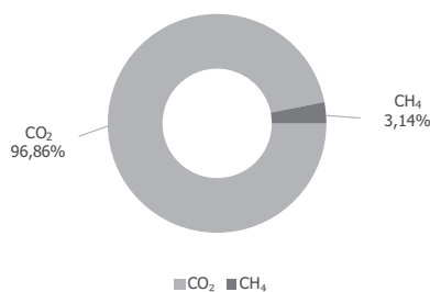
Gráfico 20. Contribución por tipo de GEI a las emisiones de los subgrupos del grupo CRF "Residuos". Año 2010.
