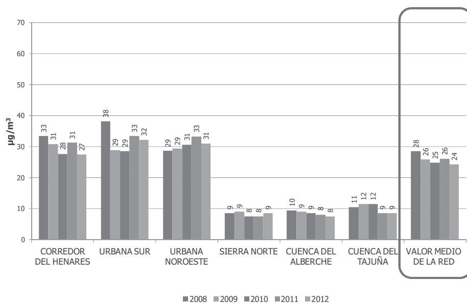
Gráfico 4. Comparativa por zona de la media anual de NO 2 . Periodo 2008-2012
