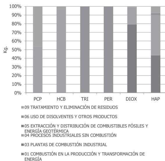
Gráfico 10. Emisiones de COP del sector industrial. Año 2010.
