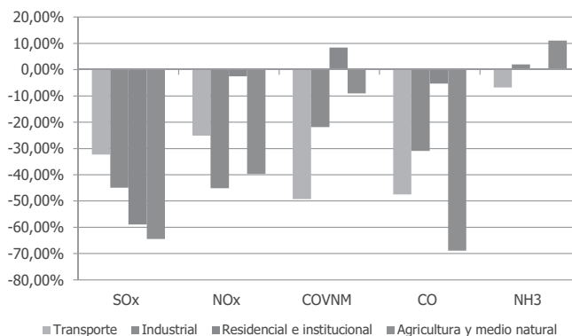
Gráfico 12. Tendencias acumuladas de las emisiones de sustancias acidificadoras y precursoras del ozono. Período 2005-2010.
