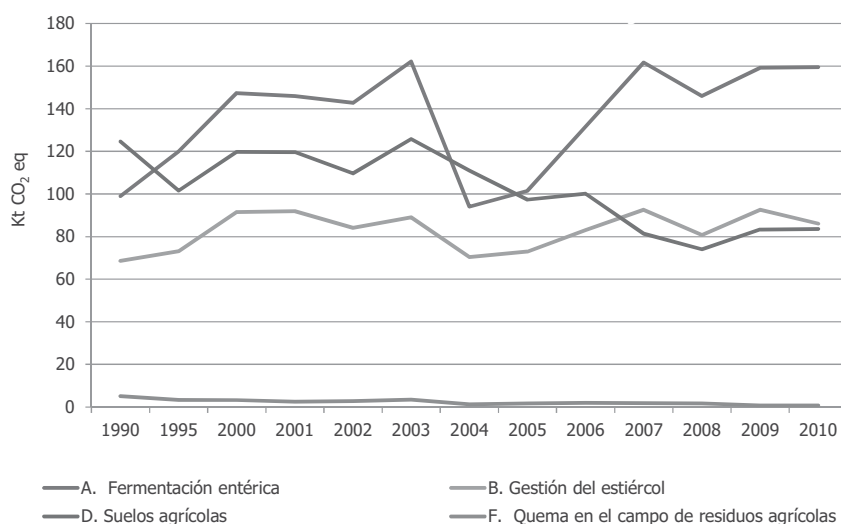
Gráfico 11. Evolución de las emisiones de GEIs del grupo CRF "Agricultura". Años 1990, 1995 y 2000-2010.
