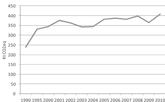
Gráfico 9. Evolución de las emisiones de GEI del grupo CRF "Uso de disolventes y otros productos". Años 1990, 1995 y 2000-2010.
