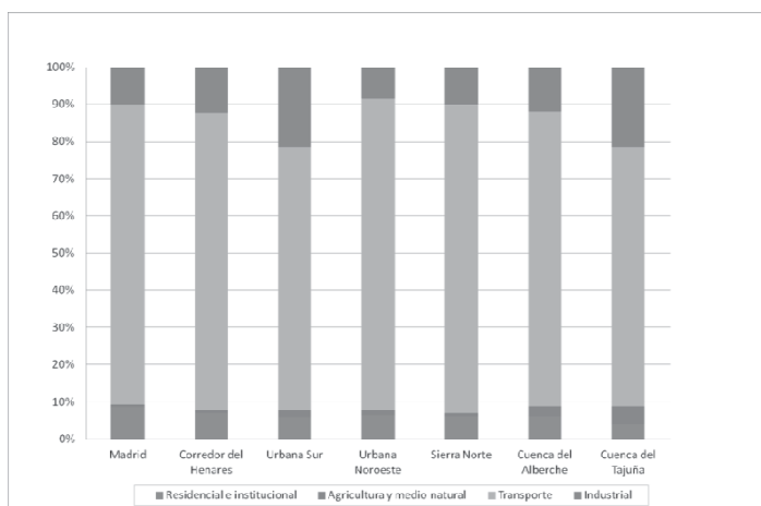
Gráfico 28. Resultados del análisis de contribución de fuentes en las diferentes zonas de calidad del aire para los niveles de CO máx 8-h.
