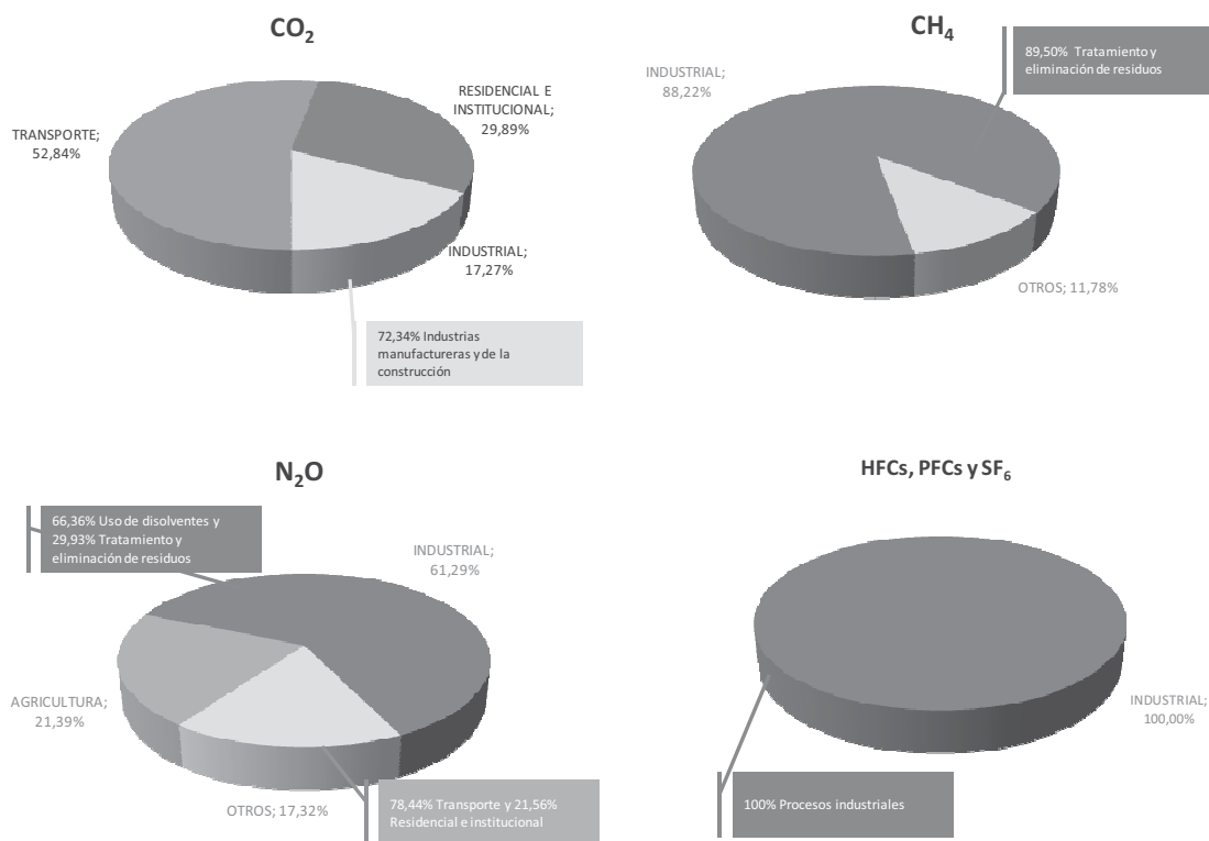
Gráfico 39. Análisis de contribución por sectores a las emisiones de GEIs. Basado en Inventario 2010.
