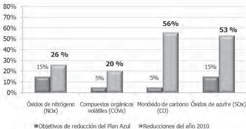
Gráfico 2. Cumplimiento de los objetivos de reducción de contaminantes atmosféricos en la Comunidad de Madrid.
