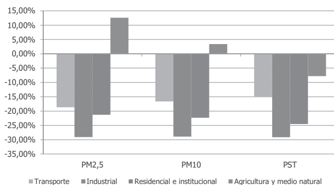
Gráfico 20. Tendencias acumuladas de las emisiones de partículas. Periodo 2005-2010.
