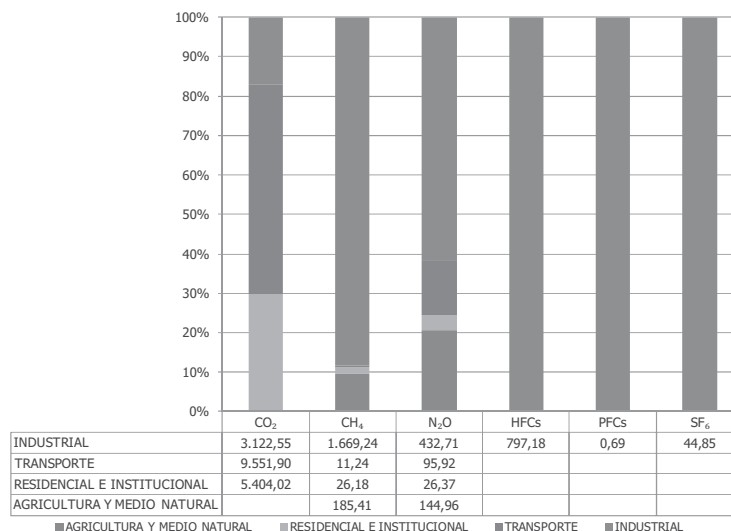
Gráfico 37. Contribución por tipo de GEI a las emisiones de los sectores. Año 2010.
