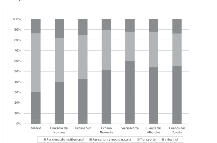
Gráfico 27. Resultados del análisis de contribución de fuentes en las diferentes zonas de calidad del aire para los niveles de PM 2,5 diario.
