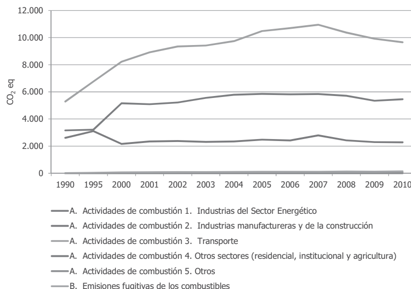
Gráfico 2. Evolución de las emisiones de GEI del grupo CRF "Energía" por subgrupo. Años 1990, 1995 y 2000-2010.
