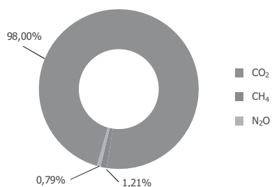
Gráfico 4. Contribución por tipo de GEI a las emisiones del grupo CRF "Energía". Año 2010.
