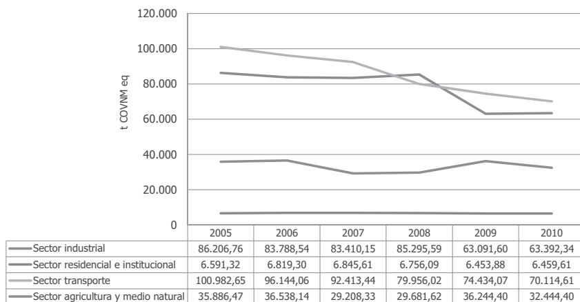
Gráfico 13. Evolución de la formación de ozono troposférico (t COVNM eq). Período 2005-2010.
