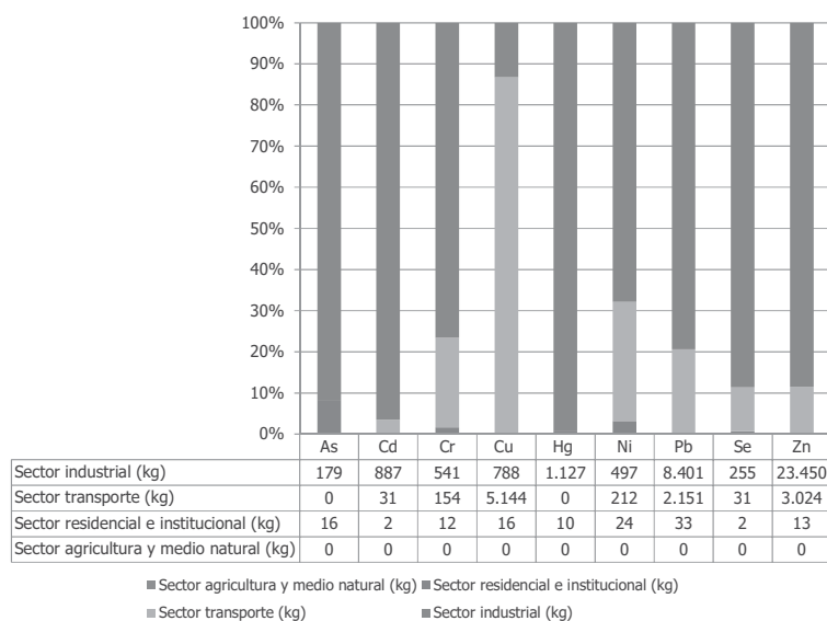
Gráfico 15. Contribución por sectores a las emisiones de metales. Año 2010.
