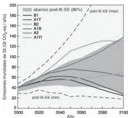
Gráfico 41. Emisiones mundiales de GEI (en Gt CO 2 -eq anuales) en ausencia de políticas climáticas adicionales para los principales escenarios entre los años 2000 y 2100. Las emisiones abarcan los gases CO 2 , CH 4 , N 2 O y CFCs
