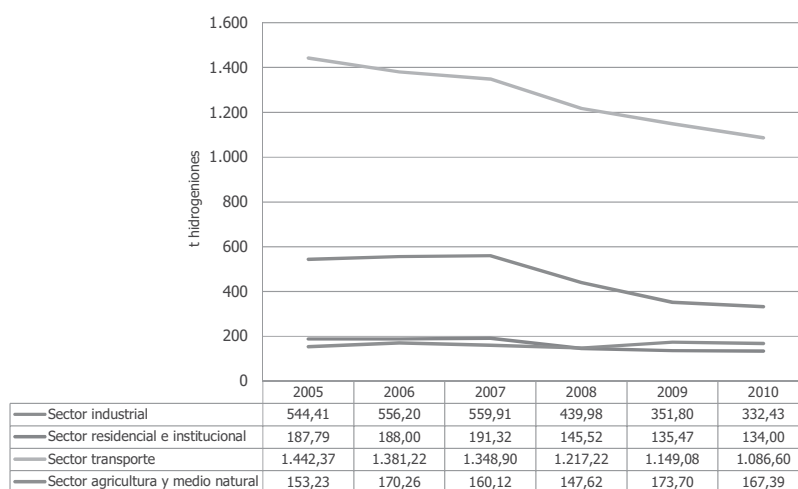
Gráfico 14. Evolución de la contribución a la acidificación (t hidrogeniones). Período 2005-2010.
