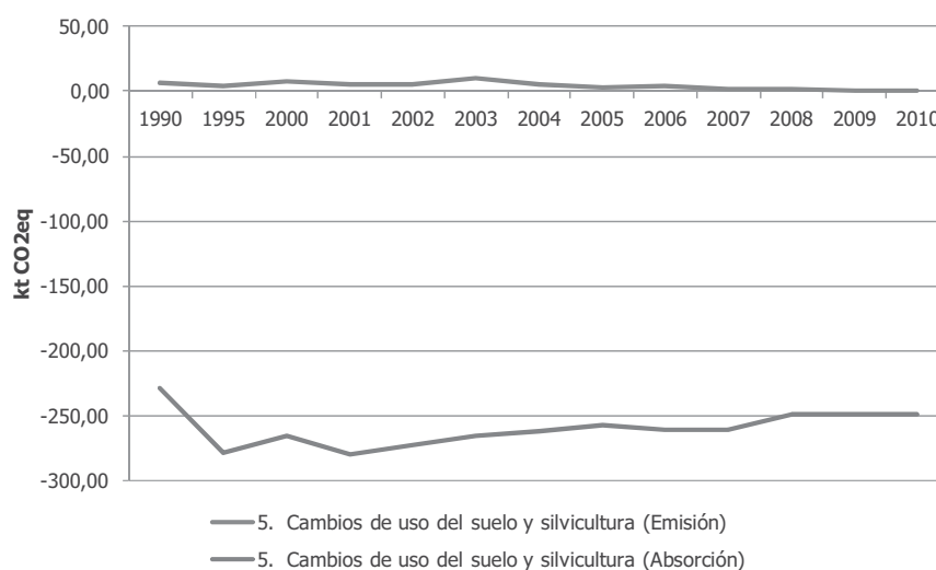
Gráfico 14. Evolución de las emisiones de GEIs del grupo CRF "Cambio de uso del suelo y silvicultura". Años 1990, 1995 y 2000-2010
