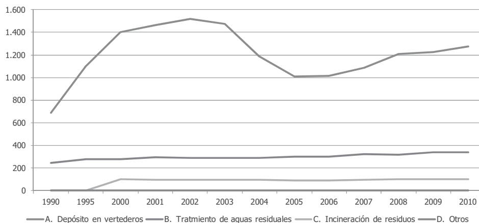
Gráfico 16. Evolución de las emisiones de GEIs del grupo CRF "Residuos". Años 1990, 1995, 2000-2010.
