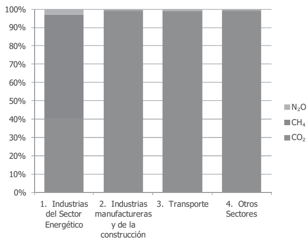
Gráfico 5. Contribución por sectores y tipo de GEI al subgrupo "A. Actividades de combustión" (Grupo CRF "Energía"). Año 2010.
