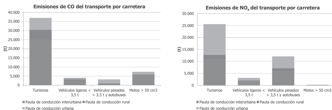
Gráfico 19. Contribución de las diferentes tipologías de vehículos, en función de la pauta de conducción, a las emisiones de NO x y CO. Año 2010.
