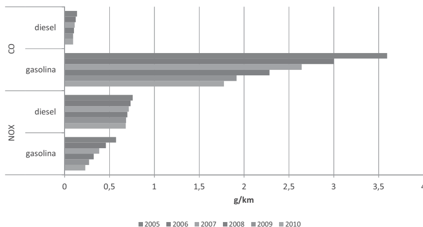
Gráfico 17. Factores de emisión medios por kilómetros para turismos a nivel nacional. Periodo 2005-2010.
